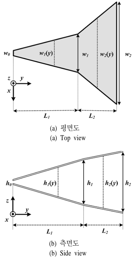
그림 1. TEM 혼 안테나의 기본 구조 Fig. 1. The basic structure of the TEM horn antenna.
