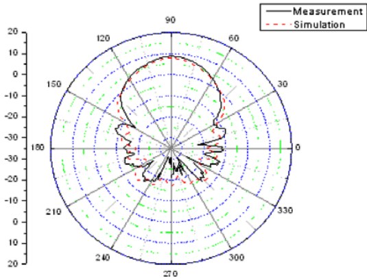
(d) H-평면 복사 패턴(3.5 GHz) (d) H-plane radiation pattern(3.5 GHz)
