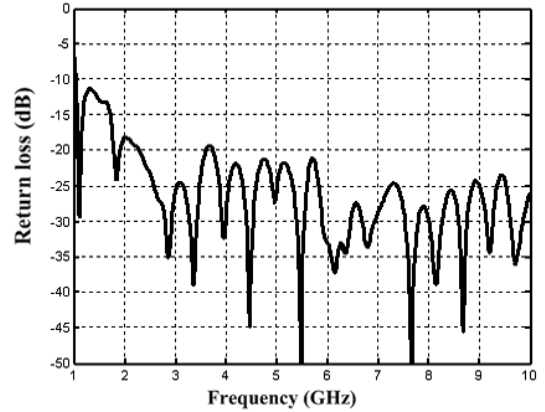
그림 3. TEM 혼 안테나 시뮬레이션 반사 손실
