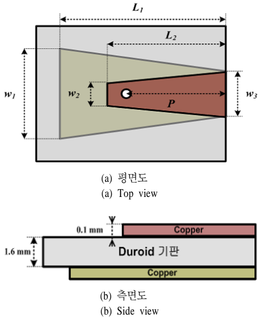
그림 4. 밸런의 기본 구조 Fig. 4. The structure of the balun.
